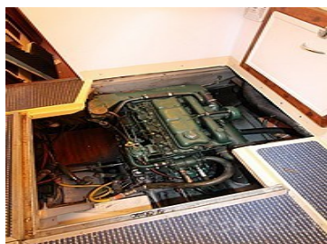
Moteur tribord
